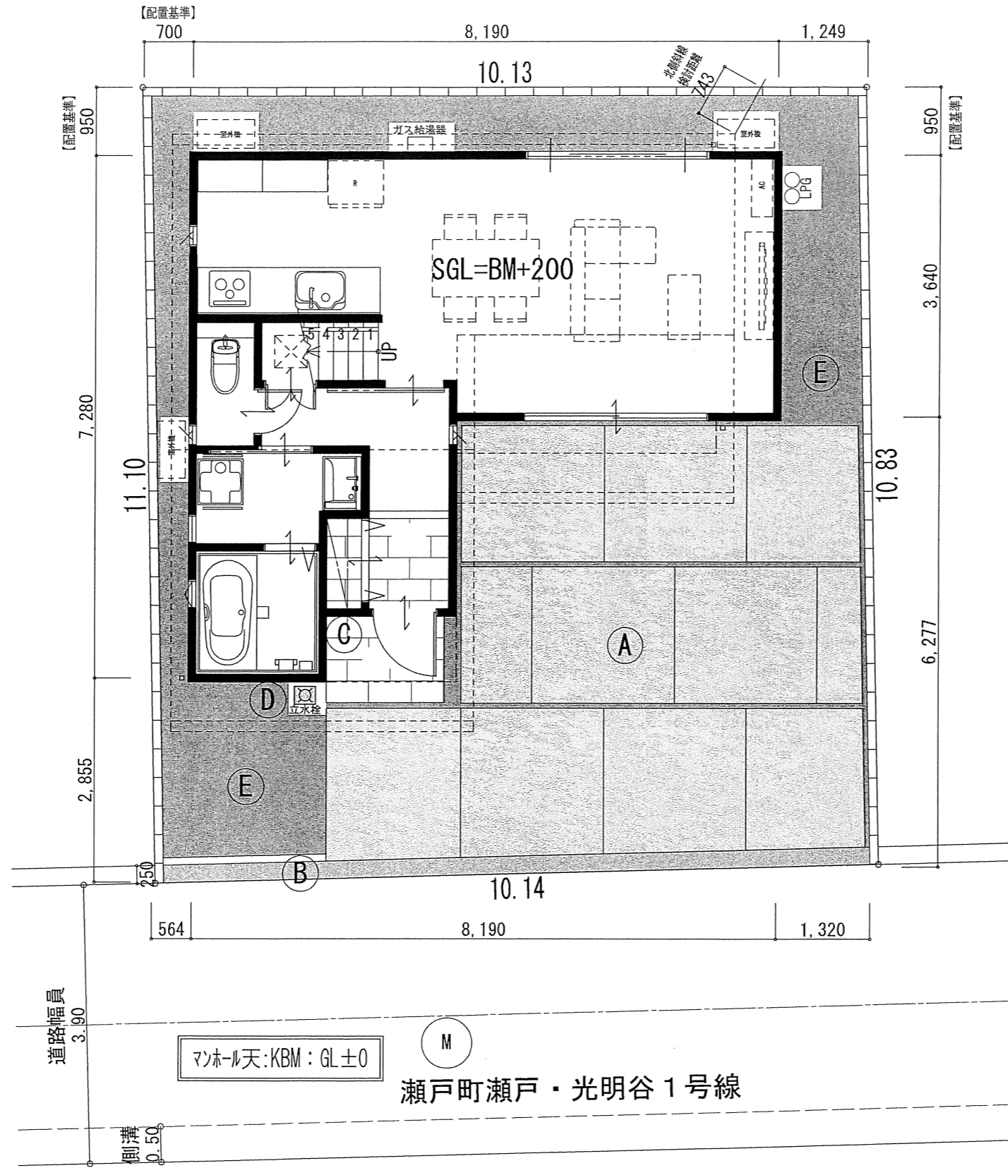
配置図 S: 1/75
