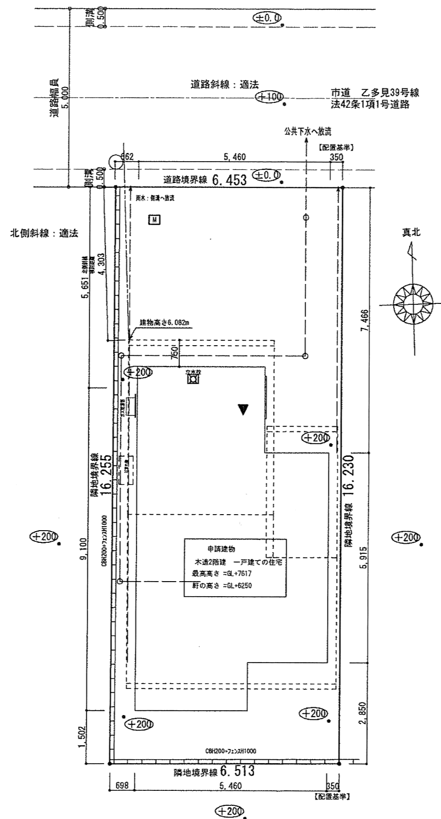
配置図 S:1/100
