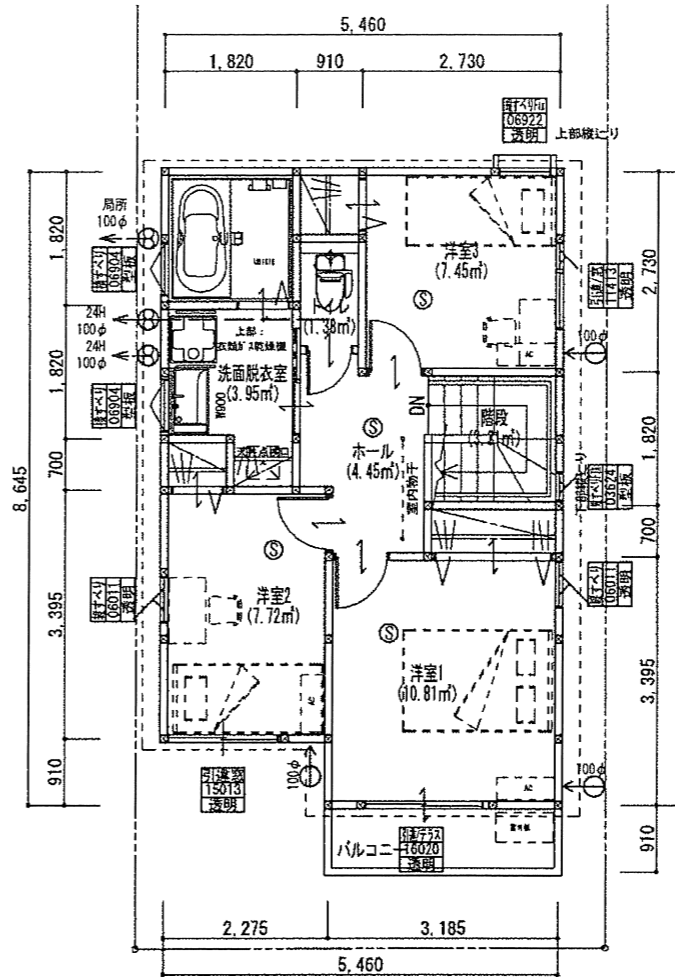
2階平面図 S:1/100
