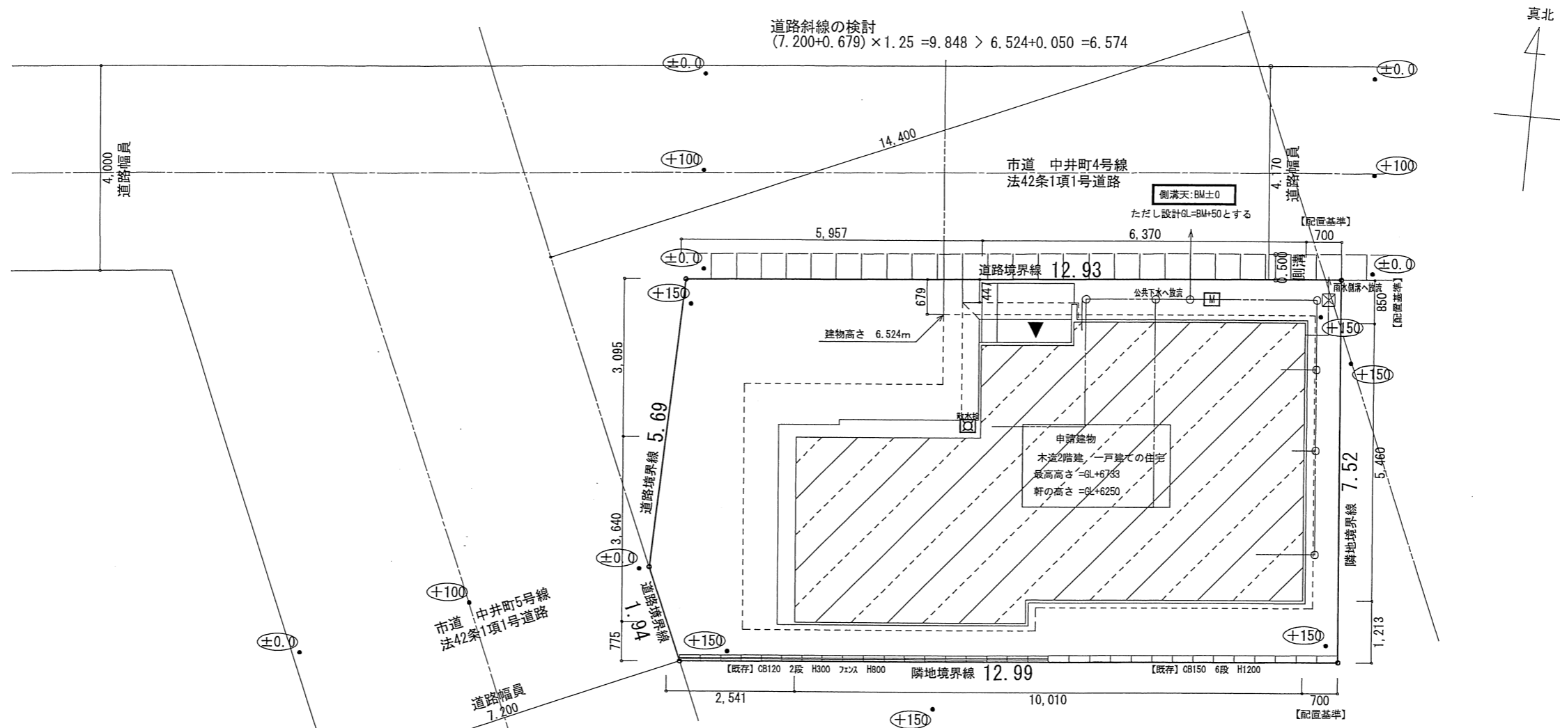
配置図 S:1/100
