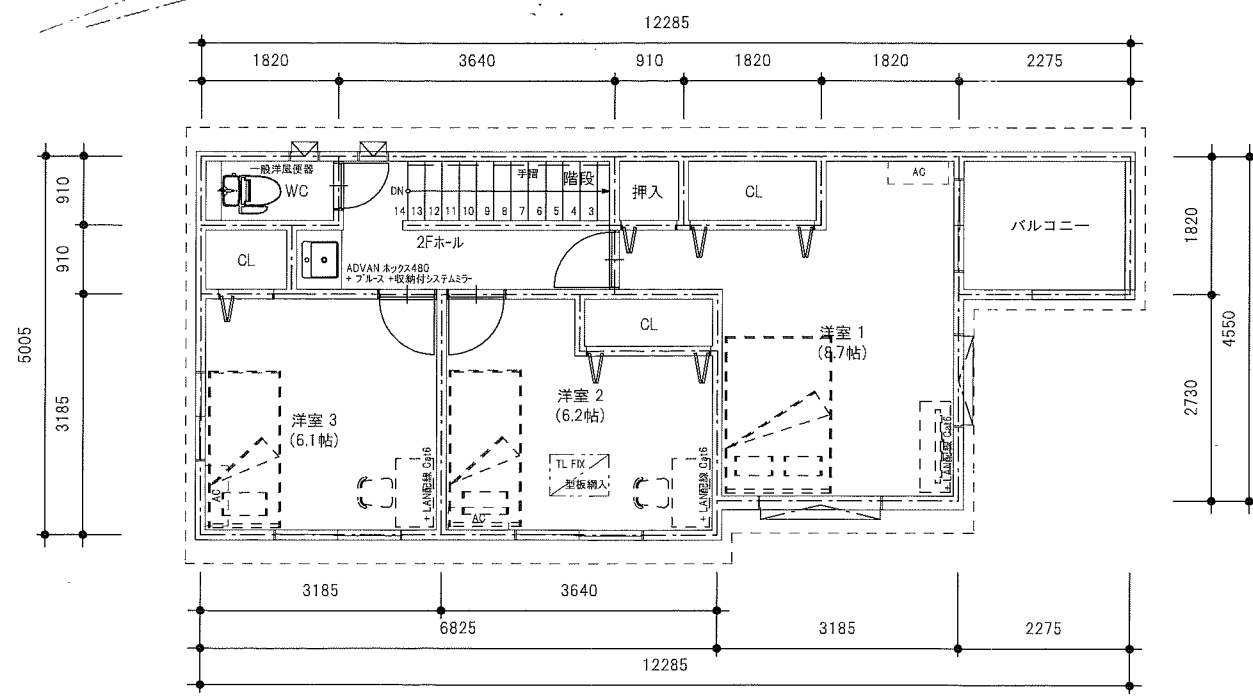
2階平面図
